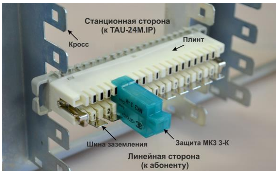
Рисунок 9 – Схема подключения
