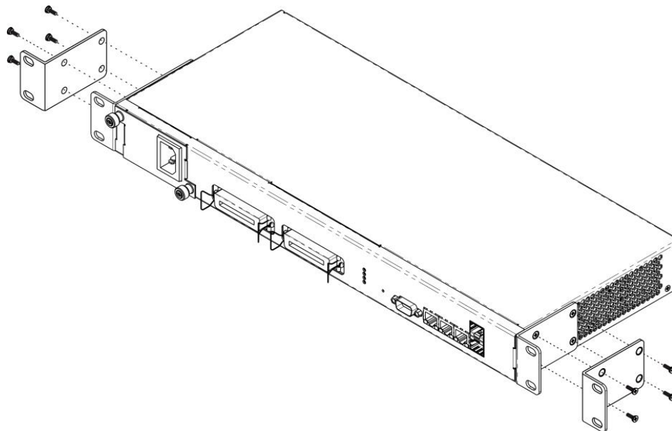
Рисунок 10 – Крепление кронштейнов
